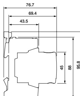
OVR T2 4L 40-275s P TS QS OVR T2 4L 80-275s P TS QS
